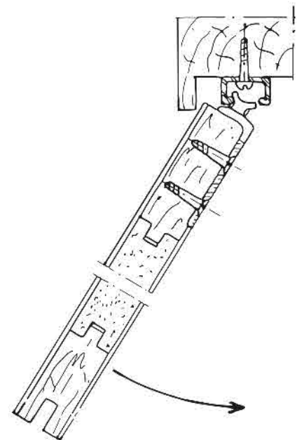
COUPE DE PORTE EQUIPEE DE PATINS MINITUB SECTION DOOR USING MINITUB SLIDER SCHNITT DURCH DIE MIT MINITUB AUSGERÜSTETEN TÜREN SECCION DE UNA PUERTA CON PATIN MINITUB
