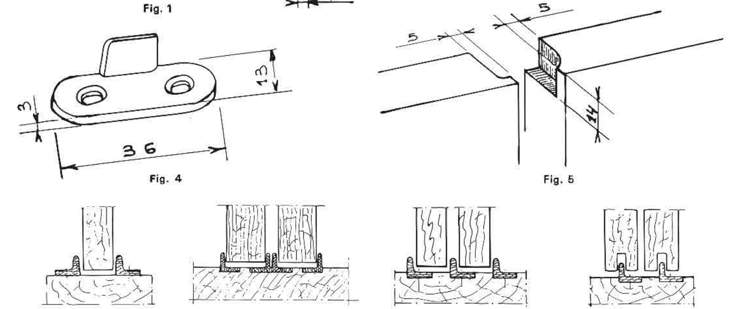
Fig. 1 : Détail Patin Réf. 111 Nr. 1 : Top slider Nr. 111 detail Abb. 1 : Detail des Gleiters Nr. 111 Fig. 1 : Detalle del patin 111. Fig. 2 : Fixation du rail Nr. 2 : Track fixing. Abb. 2 : Laufschienebefestigung Fig. 2 : Colocacion de la guía. Fig. 3 : Butée Réf. 1083 Nr. 3 : Stop Nr. 1083 Abb. 3 : Anschlag Nr. 1083. Fig. 3 : Tope Ref. 1083. Fig. 4 : Guide du bas Réf. 1123 Nr. 4 : Guide Nr. 1123. Abb. 4 : Bodentführung Nr. 1123. Fig. 4 : Guía inferior Ref. 1123. Fig. 5 : Logements à faire pour la butée pour portes se rejoignant au centre. Nr. 5 : Mortise into the leaves for a door with two leaves coming together again the centre. Abb. 5 : Aufräsung für Anschlag, falls sich 2 Türen auf einer Schiene in der Mitte schließen. Fig. 5 : Es necesario hacer un corte para el tope cuando las puertas se reunen en el centro. Fig. 6 : Exemples de guidage du bas. Nr. 6 : Examples of guiding Abb. 6 : Beispiele für verschiedene Anwendungsmöglichkeiten der Bodentführungen. Fig. 6 : Ejemplos de guiado.
