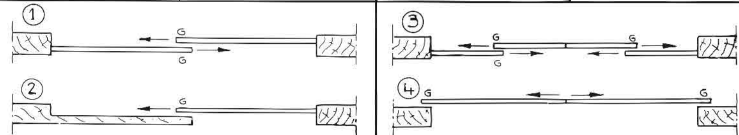
Fig. 7 : Exemples de portes réalisables avec le patin MINITUB.
