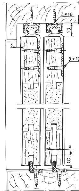
COUPE DE PORTE EQUIPEE DE PATINS MINITUB SECTION DOOR USING MINITUB SLIDER SCHNITT DURCH DIE MIT MINITUB AUSGERÜSTETEN TÜREN SECCION DE UNA PUERTA CON PATIN MINITUB
